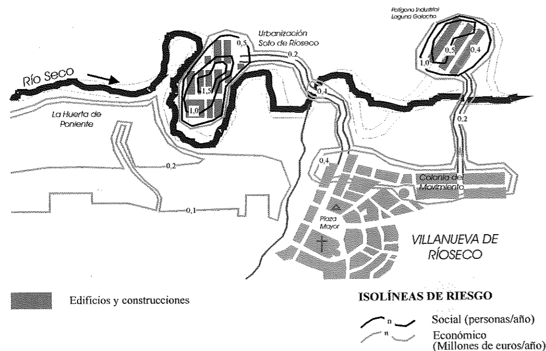
Fig. 5. Ejemplo de un mapa de riesgo de inundaciones integrado (con isóneas para el riesgo social y económico), de ámbito municipal, para el municipio idealizado de Villanueva de Ríoseco. Adaptado de Díez y Pujadas (2002).
