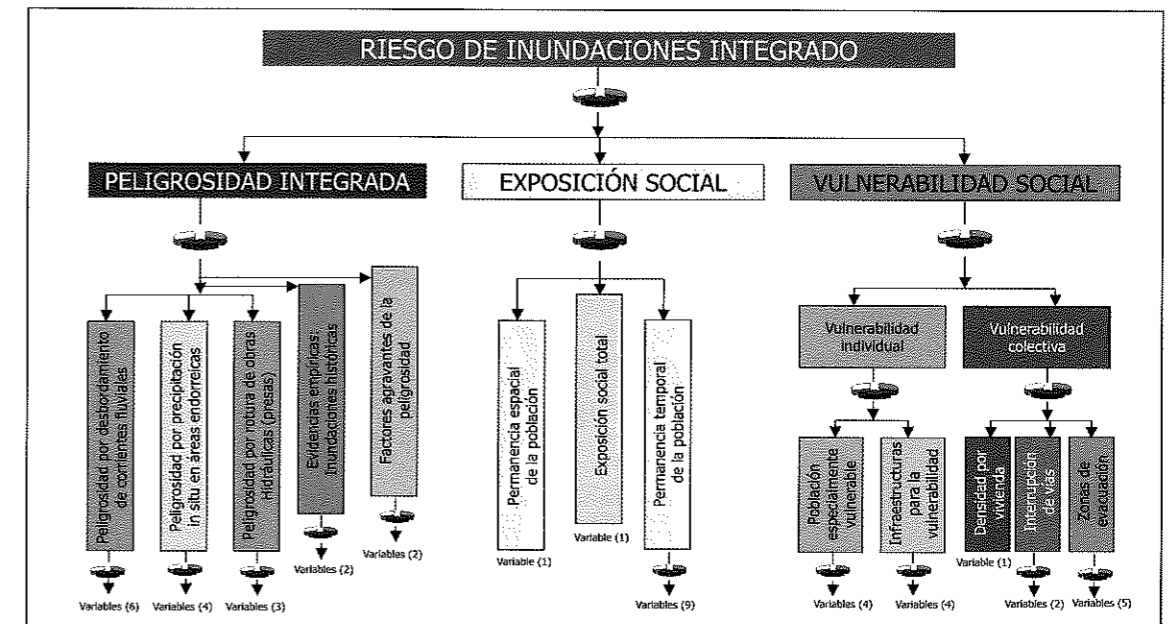
Fig. 4. Esquema metodológico sobre los sucesivos análisis y desagregaciones (símbolo del círculo partido en porciones) llevados a cabo para el análisis del riesgo social por inundaciones realizado para el Plan Especial de Protección Civil ante el riesgo de inundaciones de Castilla-La Mancha (PRICAM; Díez et al., 2008a).
