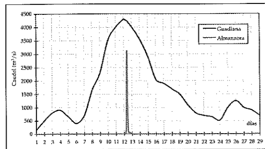
Fig. 2. Hidrogramas comparados de una crecida del río Guadiana (negro) y una avenida súbita de la rambla de Almanzora (gris). Fuente: Libro Blanco del Agua (Ministerio de Medio Ambiente, 2000).
