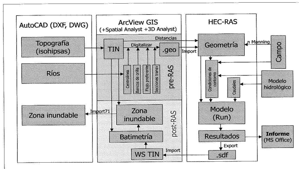
Fig. 8. Esquema metodológico para la realización del ejercicio práctico de delimitación de zonas inundables usando SIG y modelos hidráulicos.
