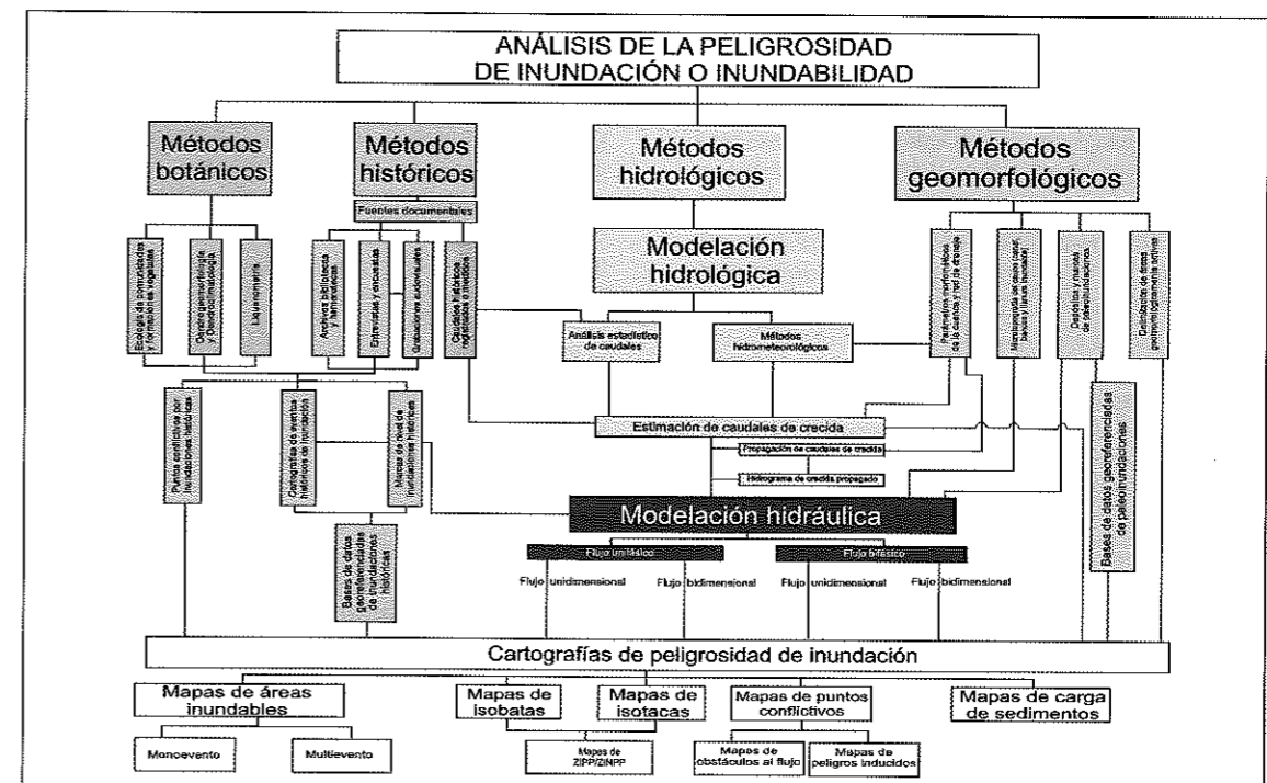
Fig. 6. Cuadro sinóptico de los diferentes grupos de métodos para el análisis de la peligrosidad de inundaciones, sus relaciones, y los tipos de cartografías resultantes (modificado y resumido de Díez, 2002). ZIPP, zona de inundación peligrosa para las personas; ZINPP, zona de inundación no peligrosa para las personas.
